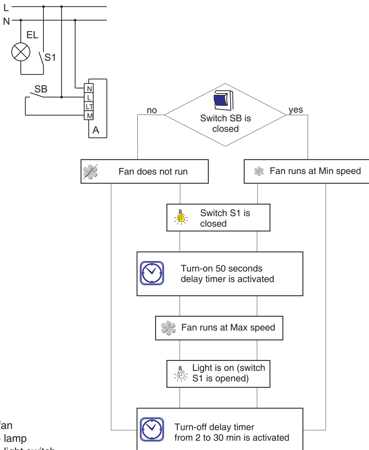
Fig. 57 wiring diagram 9
