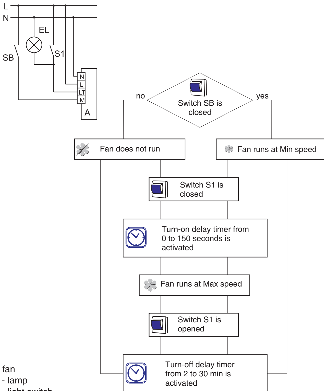
Fig. 55 wiring diagram 7
