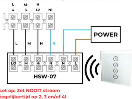
Aansluitschema Lineo aan/uit functie met HSW-07
