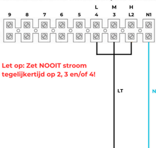
Aansluitschema Lineo aan/uit functie
